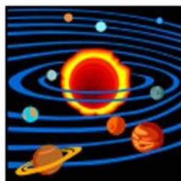
солнечная система
