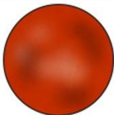
Марс
