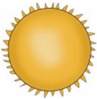
Солнце
